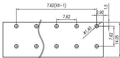
P.C.B. LAYOUT
