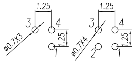
3Pin 4Pin PCB Layout
